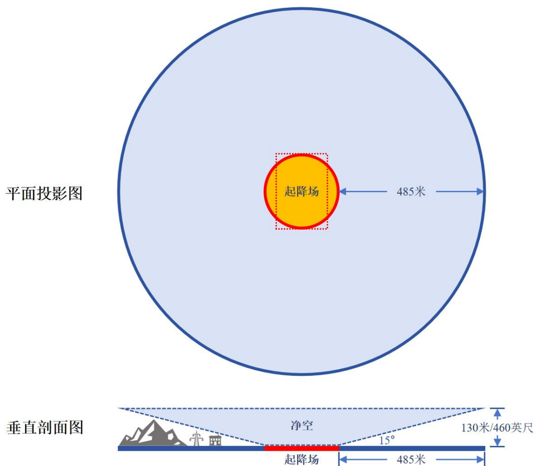
飞艇临时起降场地净空图例
